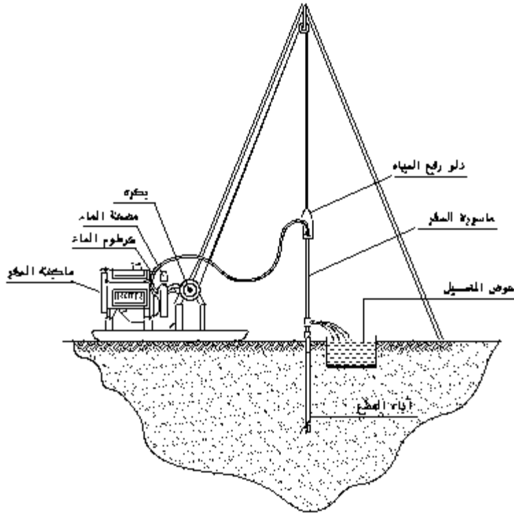
شكل رقم (3) طريقة الحفر بالاجتراف
