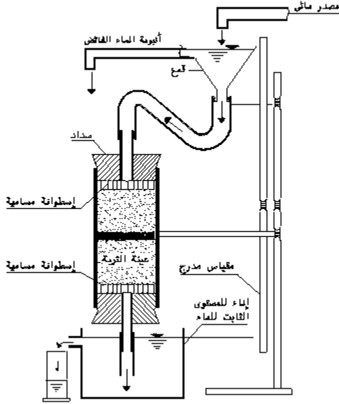
شكل رقم (14أ) جهاز إختبار النفاذية - المستوى الثابت
