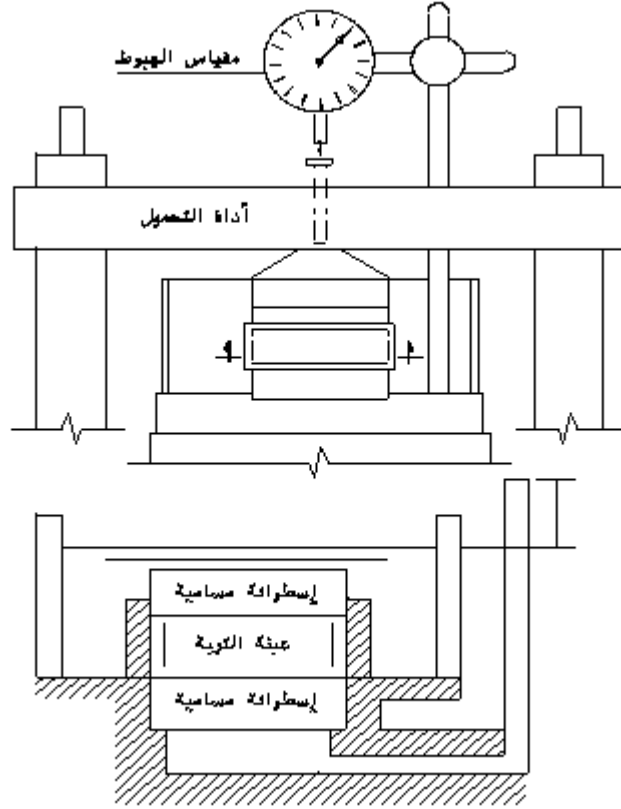
شكل رقم (13) جهاز اختبار الاندماج
