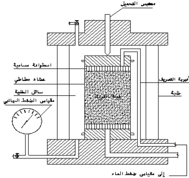
شكل رقم (12) جهاز اختبار الضغط ثلاثي المحاور
