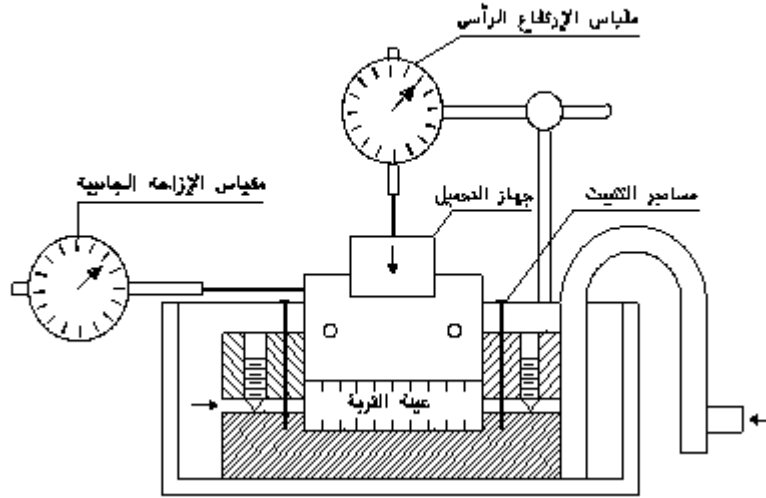
شكل رقم (9) جهاز اختبار قوة القص المباشر
