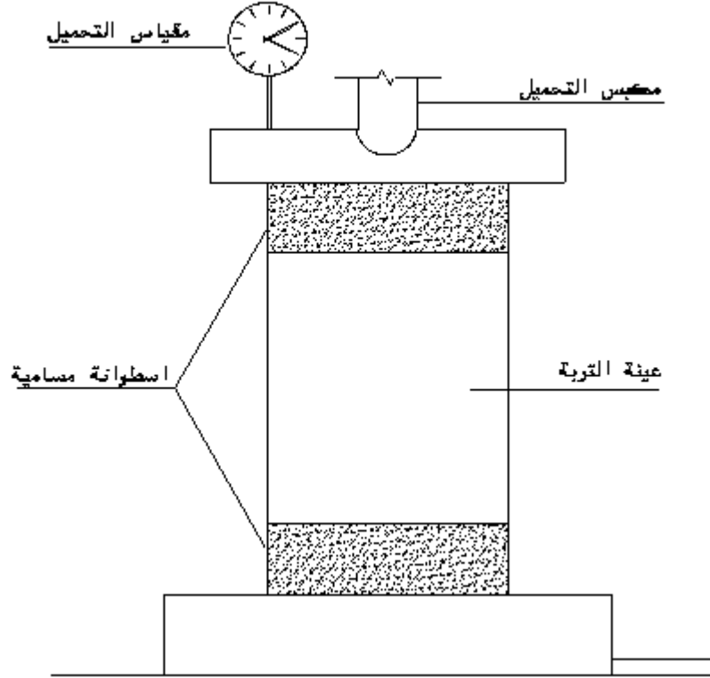
شكل رقم (11) جهاز اختبار الضغط غير المقيد
