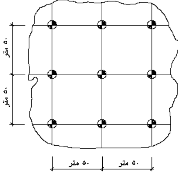
شكل رقم (4) طريقة توزيع الجسات
