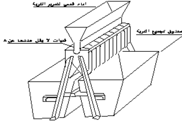
شكل رقم (7) صندوق التقسيم
