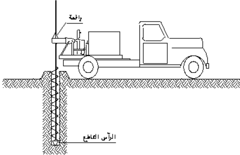
شكل رقم (2) طريقة الحفر بالمتقاب
